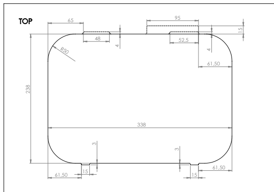
Bänkskivans uppifrån
