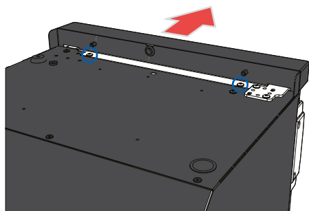
FIG.1 - RIMOZIONE MASCHERINA MASK REMOVAL
