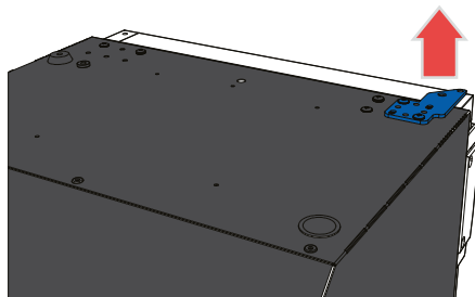
FIG.2 - RIMOZIONE CERNIERA PORTA DOOR HINGE REMOVAL
