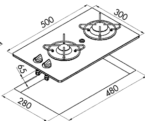
70559 2,80 kW
