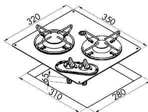
70561 2,80 kW 1 Semi Rapid-brænder (1800 W) 1 ekstrabrænder (1000 W)
