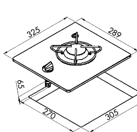
70557 1,80 kW 1 Semi Rapid-brænder (1800 W)
