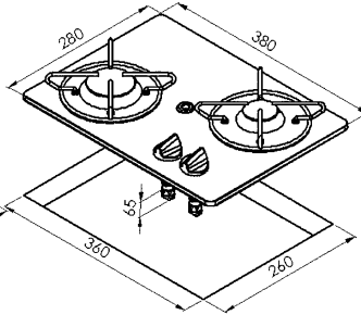
70558 2,80 kW 1 Puolikovapoltin (1800 W) 1 apupoltin (1000 W)
