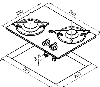
70558 2,80 kW 1 Semi Rapid-brænder (1800 W) 1 ekstrabrænder (1000 W)
