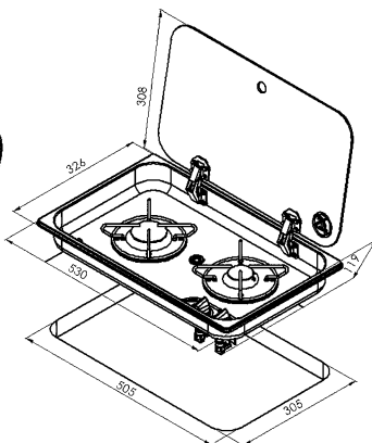
70567 2,80 kW
