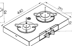
70563 2,80 kW 1 Semi Rapid-brænder (1800 W) 1 ekstrabrænder (1000 W)
