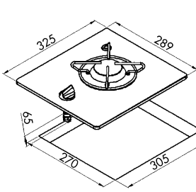
70557 1,80 kW 1 puolikiinteä poltin (1800 W)
