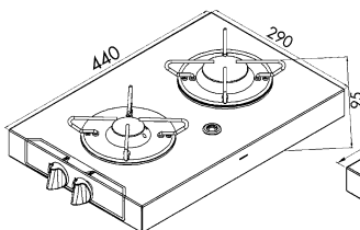
70562 2,80 kW 1 Semi Rapid-brænder (1800 W) 1 ekstrabrænder (1000 W)
